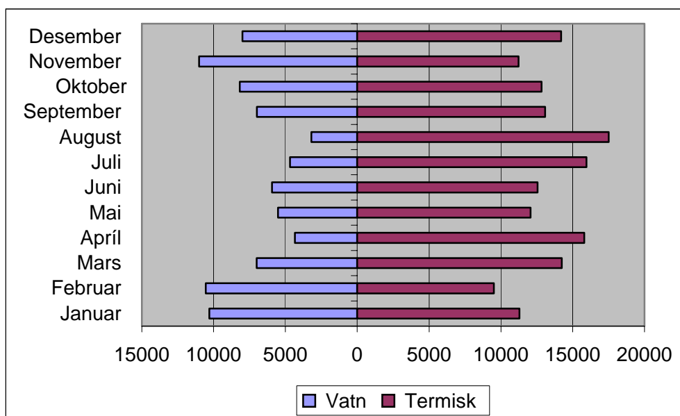
Mynd 3: Myndin vísir orkuframleiðsluna í MWh frá vatni og motorum í 2003
