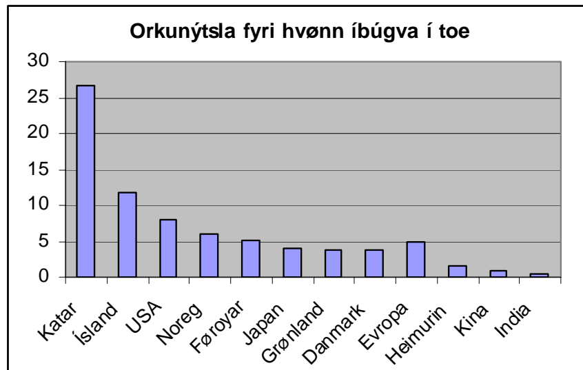
Mynd 2: Orkunýtsla fyri hvønn íbúgva í toe. Orkunýtlan í Føroyum fyri hvønn íbúgva er á leið tann sama sum fyri Evropa, men tó umleið 40% hægri enn í Danmark. Hetta, tí okkara høvuðsvinna, fiskivinnan, er sera orkukrevjandi
